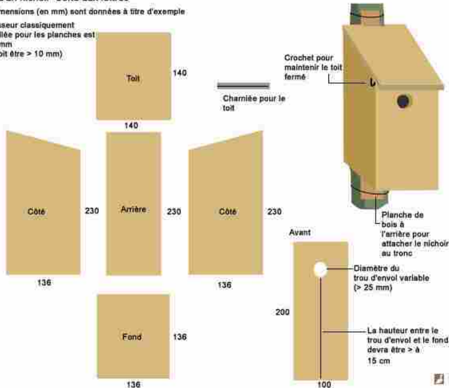
Plan d'un nichoir "boîte aux lettres"
